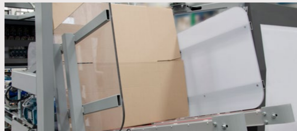
Magazzino cartoni riempibile con macchine in funzione in posizione ergonomica ed accessibile per il carico e facile cambio formato
