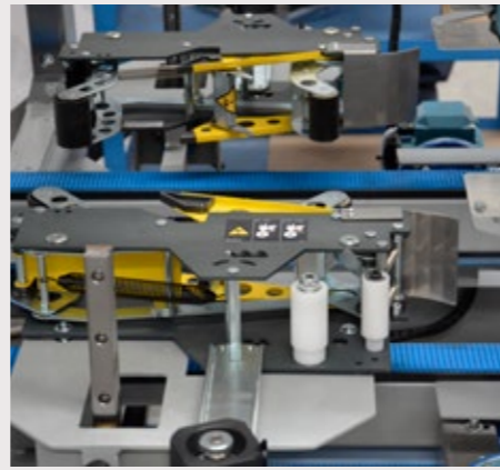
Fermeture avec du ruban ou par colle thermofusible, facilement réglable
