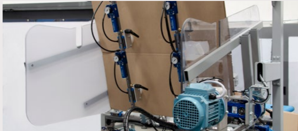
Ouverture du carton assurée par le système à ventouse
