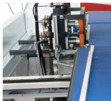
Distancia entre rueda de soldadura y producto reducida. Reducción de 10 cm de film para la producción.
