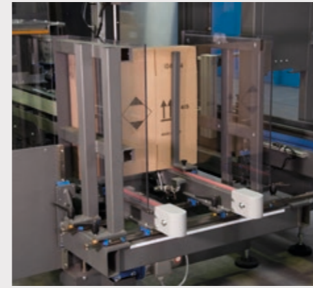
Sistema de apertura cajas en línea o a 90°. Carga de cajas facilitada gracias al almacén muy accesible. Dimensiones reducidas y óptima operatividad.
