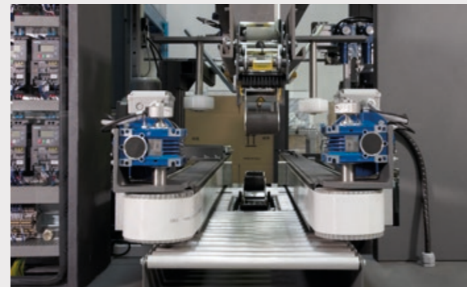
Estación de salida con correas de guía regulables desde panel según la medida de la caja.
