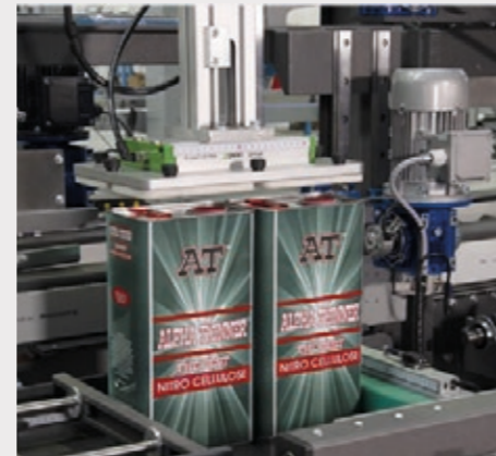
Pick & place para una toma rápida y precisa de los productos que llegan de la cinta transportadora de carga y un llenado preciso.
