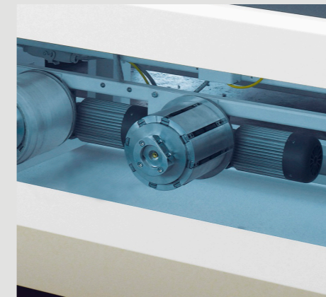
Doppia porta bobina per bobine di cartone. Optional: maniglie su bobina.
