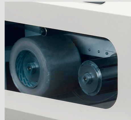
Doppio porta bobina di nastro adesivo.
