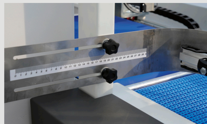
Veloce cambio formato con righe metriche.
